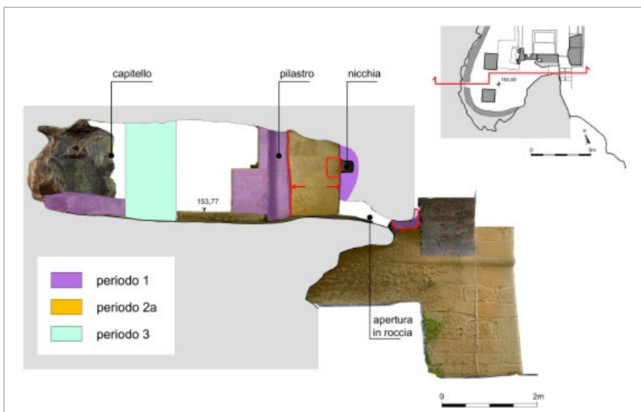
fig. 5 – Brembate, San Vittore. Sezione ovest est della chiesa rupestre in corrispondenza del presbitero.
