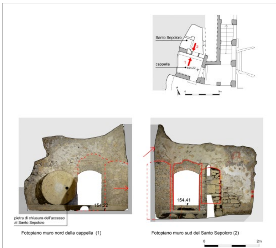
fig. 13 – Brembate, San Vittore. Ambienti a nord dell'atrio.
