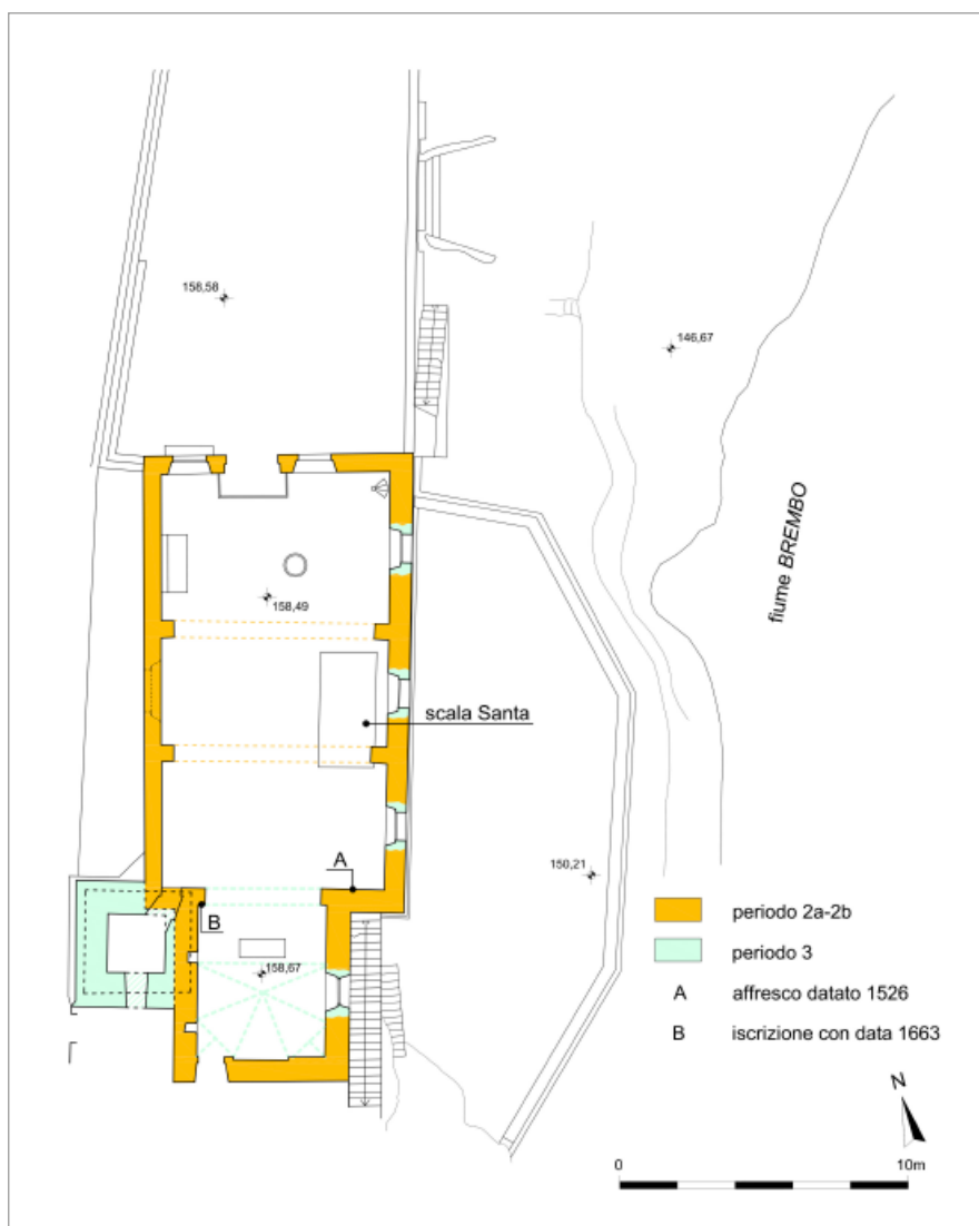
fig. 14 – Brembate, San Vittore. Pianta della chiesa superiore.
